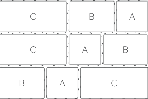
Układ kostek w warstwie
