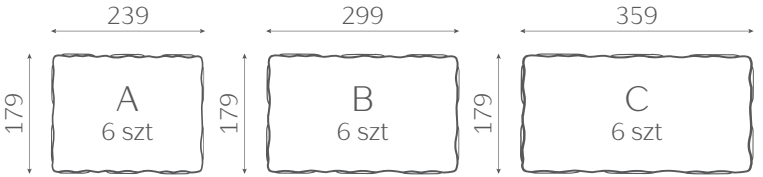
Wymiary kostki brukowej DREWBET® TROTUAR MF 60
