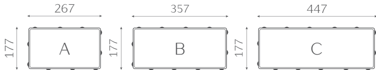
Wymiary kostki brukowej DREWBET® MIAMI MF 60
