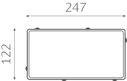
Wymiary kostki brukowej DREWBET® HOLLAND BIG MF 60
