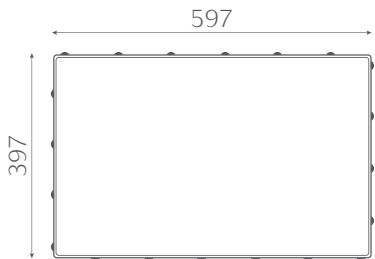
Wymiary kostki brukowej DREWBET® KORSO MF 80
