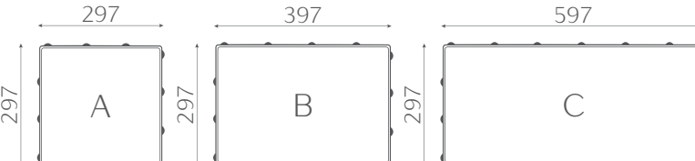
Wymiary kostki brukowej DREWBET® PORTADA MF 80
