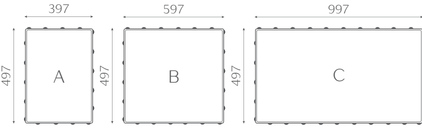
Wymiary kostki brukowej DREWBET® PORTOFINO MF 60
